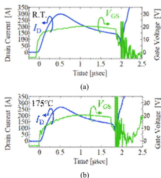
図 2. SiC MOSFET 負荷短絡実測波形 (a)室温、(b)175°C
