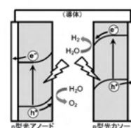
Z-scheme水分解
