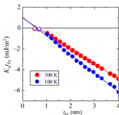
Fig. 1 Fe/NiO(001)における K_u t - t プロット。傾きがバルクの磁気異方性を、 y 切片が界面磁気異方性を表す。
