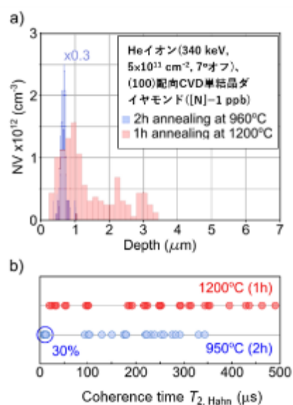
図 3. (a) 200 個及び 150 個の単一 NV センターの位置測定から得られた深さ分布, (b) コヒーレンス時間分布
