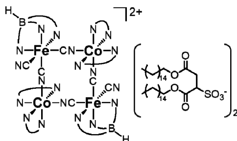
図 1 \mathbf{1}(\text{BE}_{16})_2 の構造
