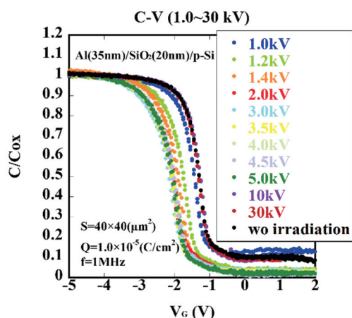
図 1 電子線照射前後の C-V 曲線
