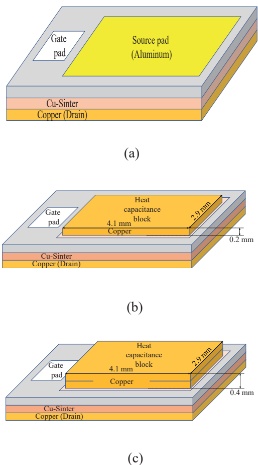
図 3 SiC MOSFET 構造図 (a)Type I,(b)Type II, (c) Type III
