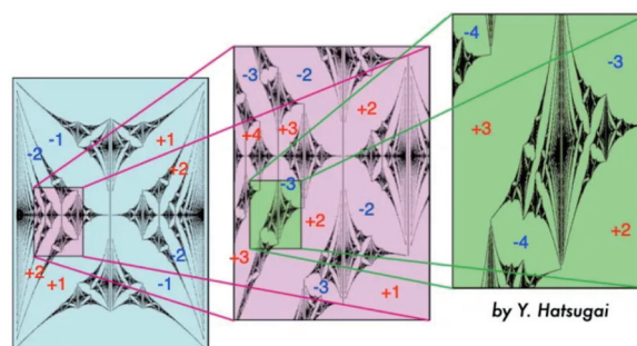
図 1 ホフスタッターの蝶と呼ばれるフラクタル構造。図の一部を拡大しても、類似の構造が次ぎ次にあらわれる。論文[2]ではこのフラクタル現象を古典的な電気回路を用いて実現した。図の数字はチャーン数と呼ばれるトポロジカル数であり、その一部は実験により具体的に決定することに成功し、エッジ状態の観測も行い、トポロジカル相の基本原理解であるバルクエッジ対応を電気回路で観測した(論文 2)。
