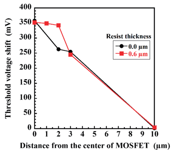
図5 閾値電圧シフトの面内距離依存性
