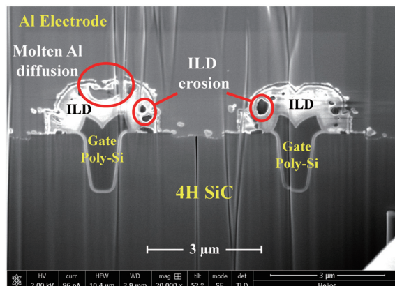
図 6. 順方向サージ電流試験による破壊後の Type I IE-UMOSFET の焼損痕から 20μm 離れた箇所の断面 SEM 画像
