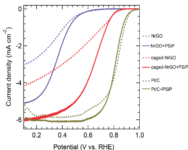
図 2. \text{O}_2 飽和 0.1M \text{H}_2\text{SO}_4 電解液中で測定した NrGO(紫色)、caged-NrGO(赤色)および Pt/C(黄色)のリニアスイープボルタモグラム。実線が \text{SiO}_2 ポリマーブラシを投入した触媒、点線が投入していない触媒の活性を表す。
