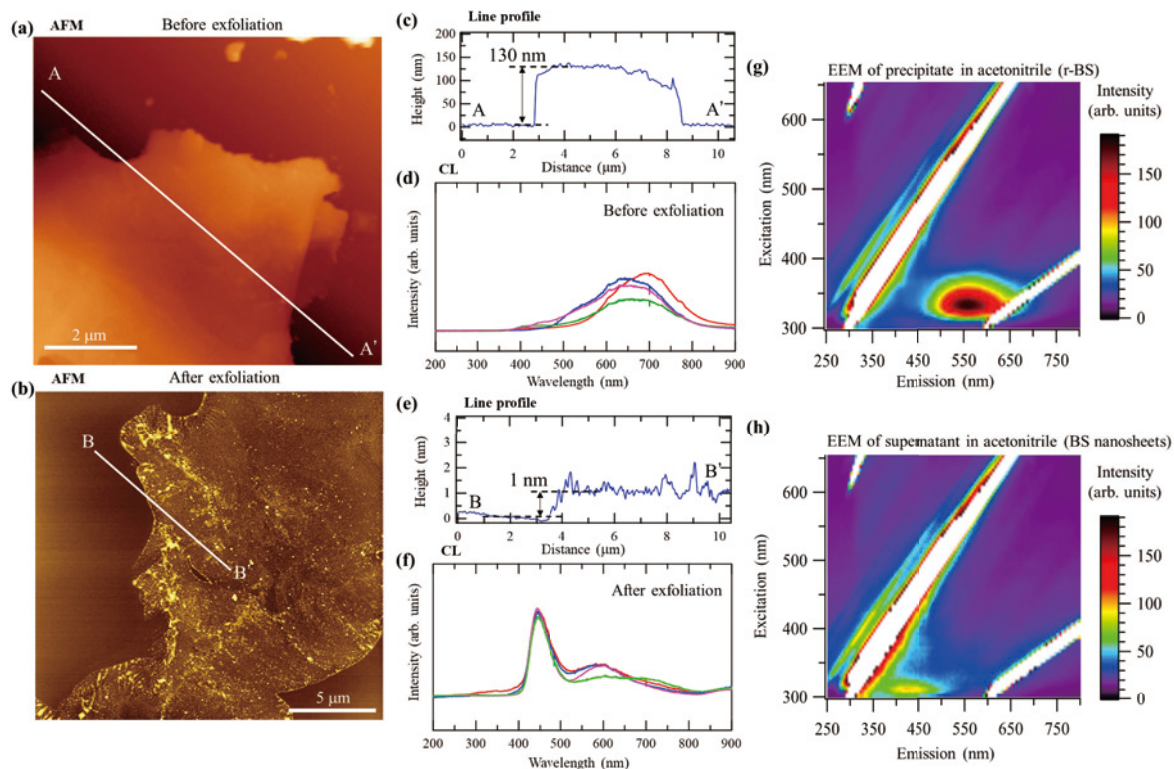
図4 (a)(b) r-BS粉末と剝離して生成したBSナノシートの原子間力顕微鏡(AFM)像 (c)(e) AFM像aとbのA-A'及びB-B'のラインプロファイル (d)(f) r-BS粉末と剝離して生成したBSナノシートのカソートルミネッセンス(CL)スペクトル (g)(h) r-BS粉末と剝離して生成したBSナノシートの励起発光マトリックス(EEMs) (J. Journal of Materials Chemistry A , 9 , 281-290 (2021).)
