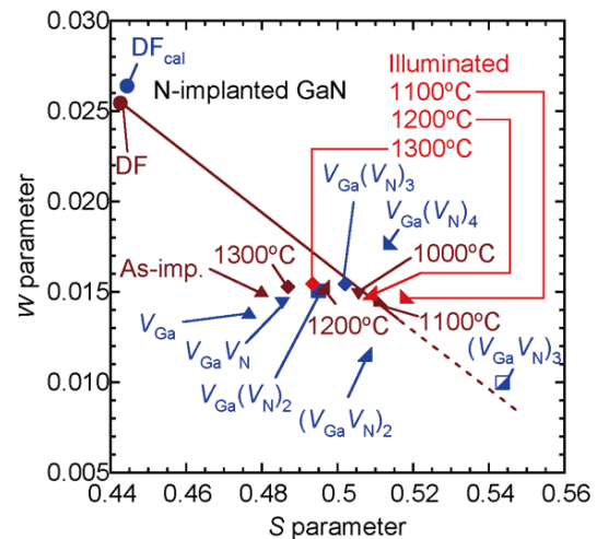
図 5. N 注入した GaN の S - \eta プロット。実験で得られた結果を赤及び茶色のシンボルで、シミュレーションにより得られた結果を青で示した。
