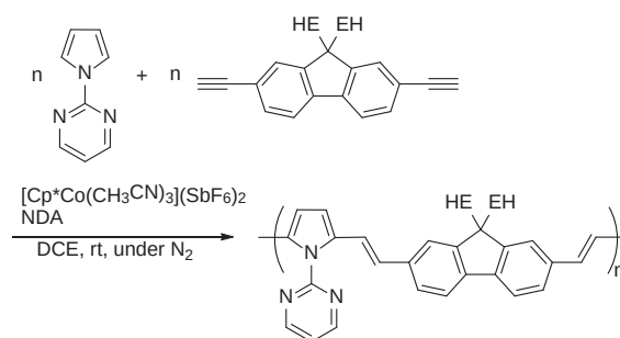
Scheme 3 アルキンのヒドロアリール化反応を利用した重付加
