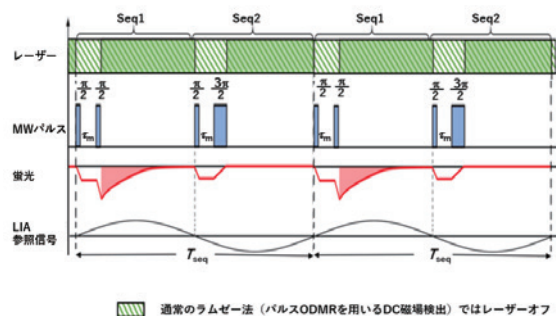
図 1 CE-Ramsey 法
