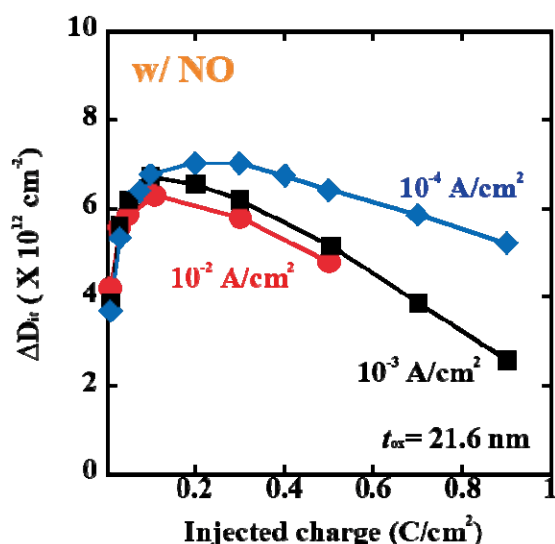
図5 界面負電荷の増加量のストレス電流密度依存性。
