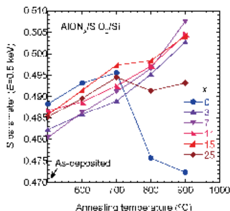
図 3. AION/ \text{SiO}_2/\text{Si} 試料について、AION 中の陽電子消滅に対応する S 値の焼鈍温度依存性。
