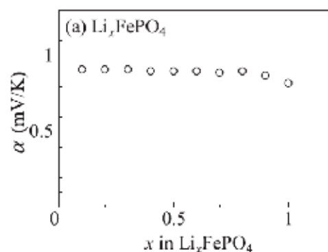
図 3 \text{LiFePO}_4 の \alpha の Li 濃度依存性
