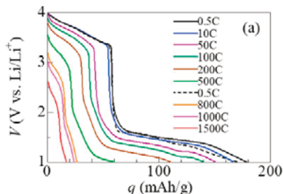
図 1 P3HT キャスト膜の高速放電
