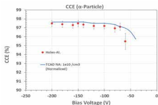
図 2.α線実験から得られた電荷収集効率のセンサーバイアス電圧依存性.実線がシミュレーションで、●が正孔の電荷収集効率である。
