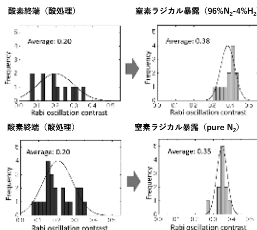
図1 窒素末端化による浅い NV センターの電荷安定化の評価にラビ振動コントラストを用いた。水素を加えない窒素ガスを用いるほうが full N 構造が増えることを示唆する結果が得られた。
