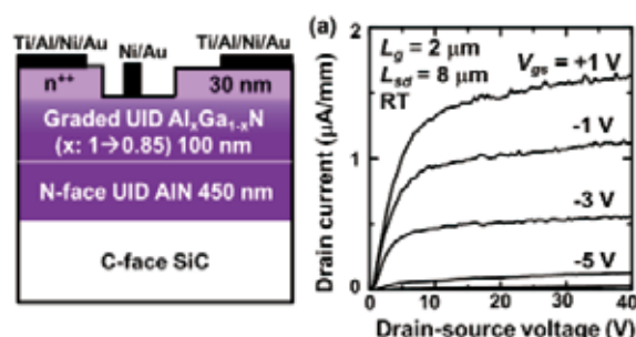
図 2: 窒素極性面 AIN-POLFET の電氣的特性
