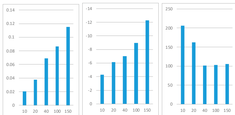
Fig.4 細孔サイズに依存する酵素吸着量 (左, 縦軸は \text{mg(enzyme)/mg(carbon)} ), 電流密度 (中, \text{mA/cm}^2 ), 酵素当たりの電流生成効率 (右, 電流密度/炭素重量当たりの酵素吸着量), 横軸は細孔サイズ (nm)
