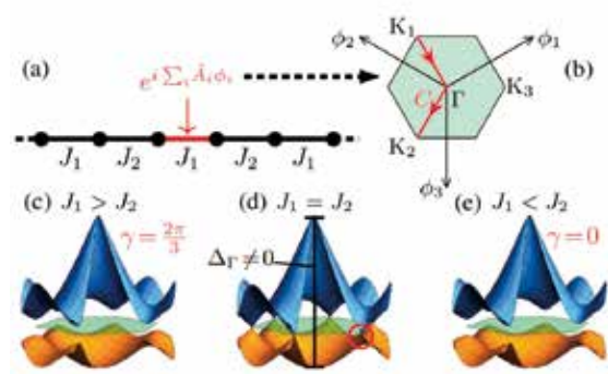
図3 (a) (b) 対称性で護られたベリー位相を定義留守ゲージ変換の概念図。(c) パラメータ空間でのエネルギーと対応する量子化ベリー位相 (論文1より引用)
