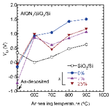
図 1. AION/ \text{SiO}_2/\text{Si} 試料のフラットバンド電圧の焼鈍温度依存性。 \text{SiO}_2/\text{Si} の結果も示した。
