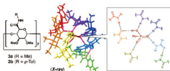
図2 アミド基を7つ導入したシクロデキストリン 3a , 3b の構造式と、(PhPO 3 H - )· 3b のX線結晶構造
