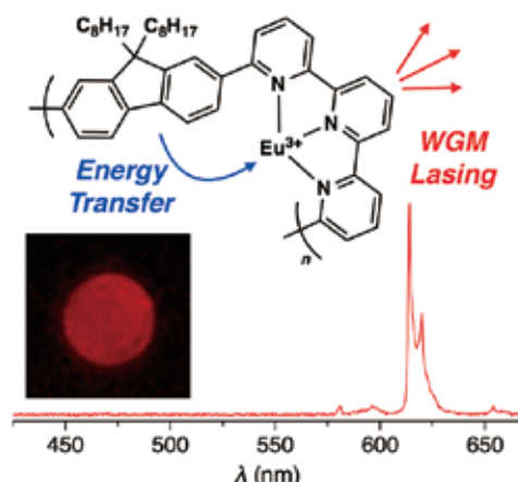
図3. フルオレン-テルピリジン交互共重合体/ユーロピウム錯体複合体からなるマイクロ球体共振器からのレーザー発振スペクトル。
