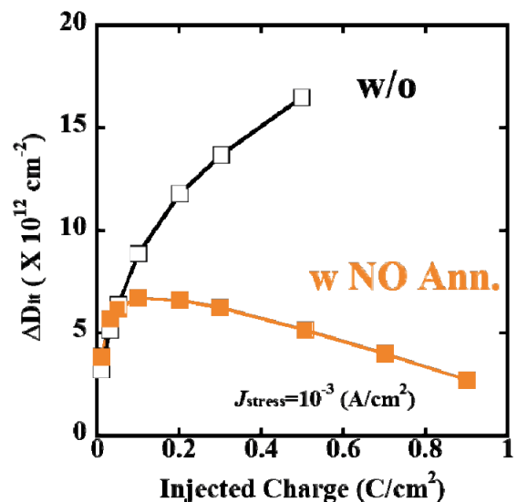
図4 ストレス印加時における界面負電荷の増加量。
