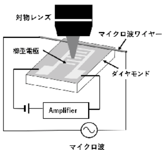
図2 単一NVセンターのスピン読み出しの光電流検出の模式図。緑色レーザー励起による2光子過程で \text{NV}^- \rightarrow \text{NV}^0 \rightarrow \text{NV}^- のサイクルを繰り返し、単位時間当たり多数発生する電子、正孔を梯型電極により捕集し、レーザーパルス列、マイクロ波パルス列を組み合わせた変調を用いてロックイン検出する。
