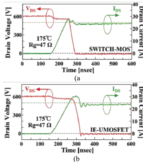
図 7 175℃での(a)SWITCH-MOS と (b)IE-UMOSFET のターンオン波形
