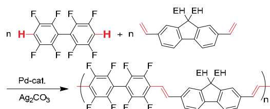
Scheme 1 直接的アルケニル化重縮合
