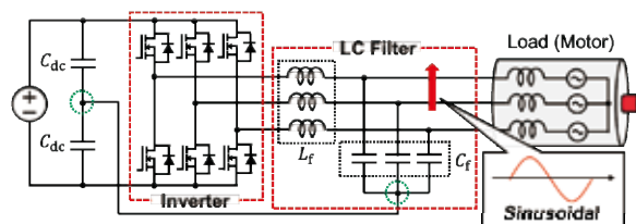
図 4 DCM を用いた正弦波電圧出力インバータ【 3 】
