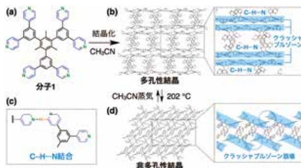
図 7. (a)分子 1 の構造 (b)多孔性結晶の構造 (c) \text{C-H}\cdots\text{N} 結合模式図 (d)孔が崩壊した後の結晶構造。
