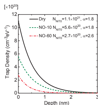
図 4 NIT 密度分布の酸化膜形成条件依存性
