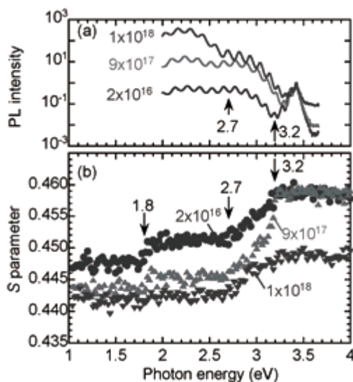
図 1. GaN-on-Si の S 値の光照射エネルギー依存性。同一試料の PL 測定の結果も示した。
