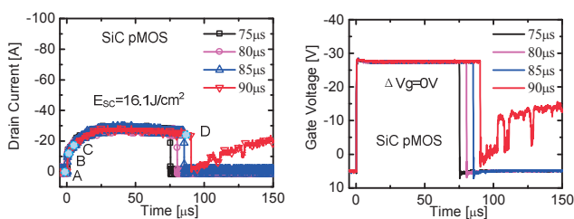
図 2 SiC p-MOSFET 負荷短絡耐量評価結果
