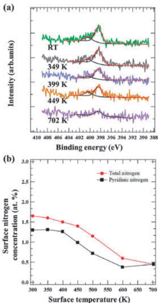
図4 (a) DA/HOPG の XPS 測定結果 (温度依存性)、(b) XPS で見積もられた窒素量およびピリジン型窒素量の温度依存性
