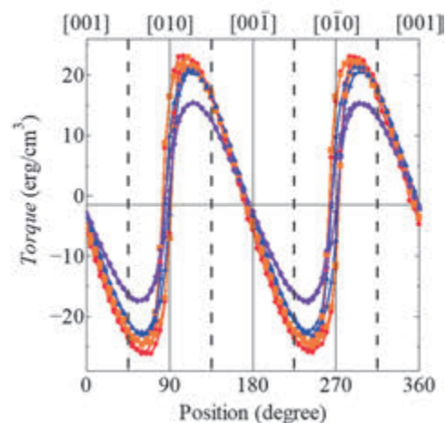
図1 MSO 上に成長した CFO(001)の磁気トルク曲線
