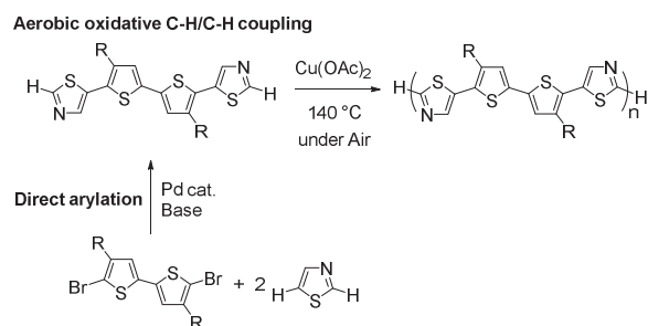
Scheme 3 銅触媒による酸素酸化重合
