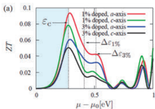
図 2-2 磁性半導体 CuFeS 2 の熱電変換性能指数とドーピング効果の理論
