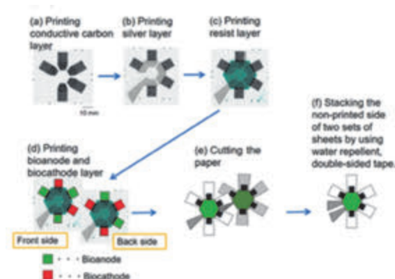
図 1・2 電池の作製プロセス
