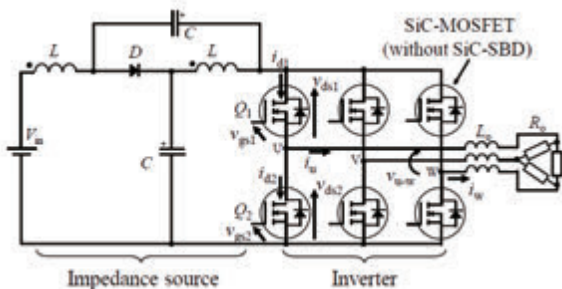
図 1・1 インピーダンスソースインバータの回路例
