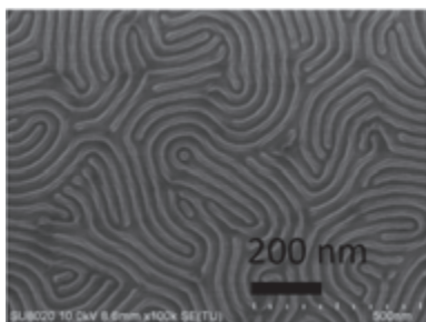
図1：PS- b -PMMA のラメラ構造を用いて形成したポリスチレンの凹凸構造。
