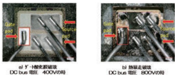
図 1 SiC n-MOSFET 破壊試験後の素子写真
