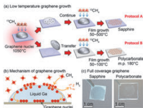
図 1-1 室温グラフェン成長模式図
