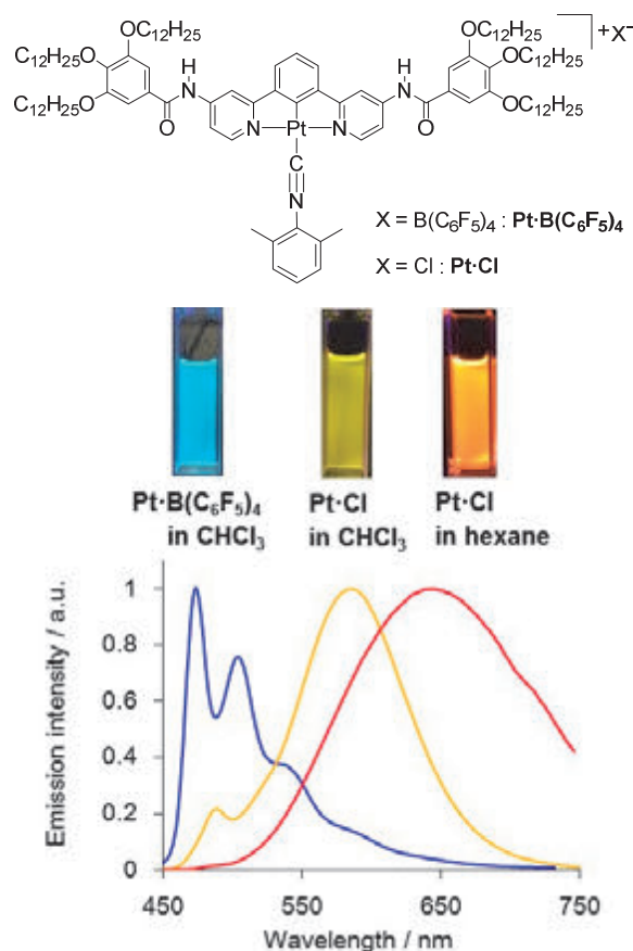
図 2 白金錯体の構造と外部環境に応じた発光
