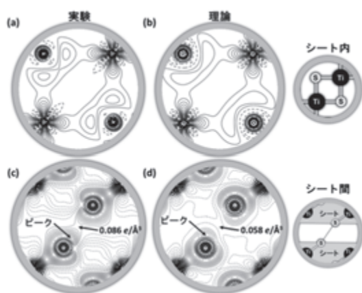
図1 図1に(a,c)実験と(b,d)理論計算で観測されたシート内およびシート間の電子分布
