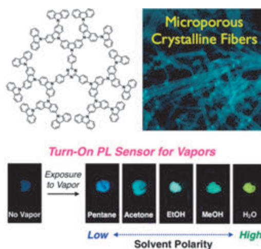
図4 \pi 共役 dendrimer の分子構造、自己組織化ポラスファイバーの蛍光顕微鏡写真、および各溶媒蒸気に晒したときの蛍光色変化。
