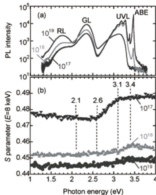
図 3. Mg 注入 GaN について 1300°C 焼鈍後の (a) 低温 PL 測定結果, 及び (b) S 値の光照射エネルギー依存性.
