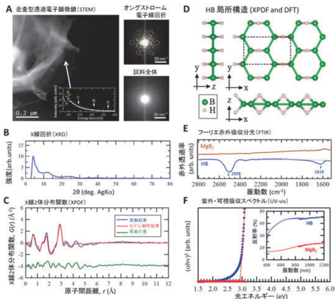
図7 ホウ化水素(HB)シートの(A)走査型透過電子顕微鏡像、電子線回折像、(B)X線回折、(C)X線2体分布関数、(D)局所構造モデル、(E)フーリエ赤外吸収分光スペクトル、(F)紫外・可視吸収スペクトル
