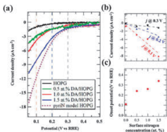
図3 (a) DA/HOPG の ORR 測定結果 (DA 分子吸着量依存性)、(b) 電流密度( j )の窒素濃度依存性、(c) ORR 開始電位 (V vs. RHE@ -1\mu\text{A/cm} ) の窒素濃度依存性
