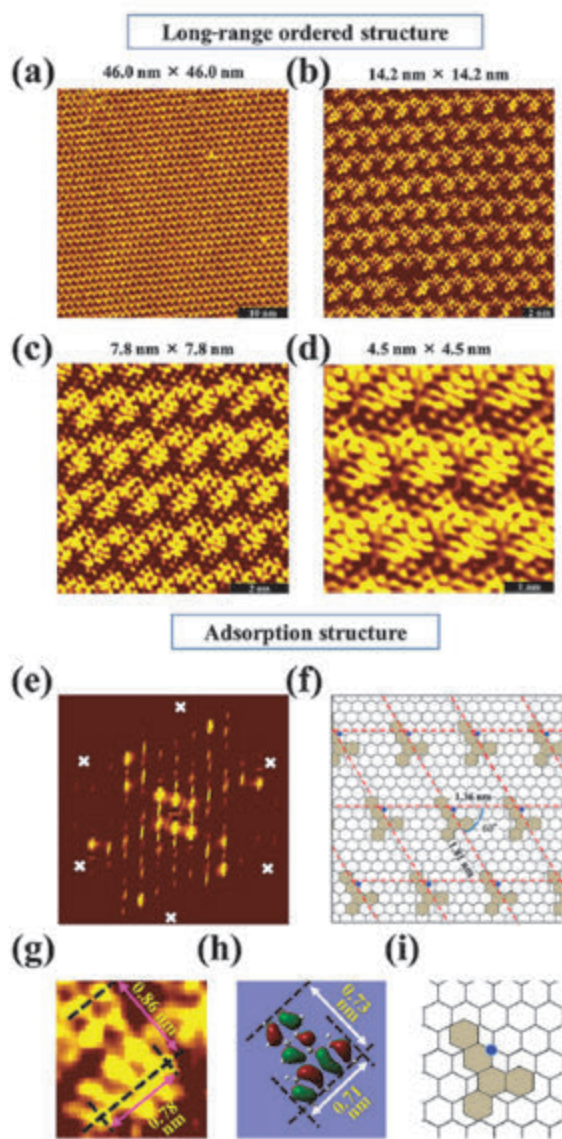
図2 (a-d)DA/HOPGのSTM像(バイアス電圧-95 meV、トンネル電流3.1 nA)、(e)STM像cのフーリエ変換像、(f)DA/HOPGの吸着モデル、(g) HOPG上のDA分子を拡大したSTM像、(h) ガウシアンで計算したDA分子のHOMOの空間分布、(i) HOPGのDA分子の吸着モデルを拡大した像
