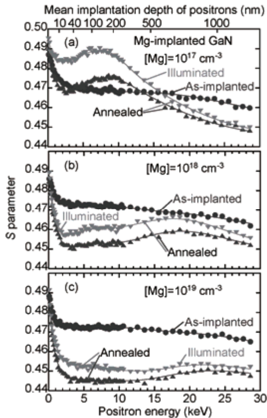
図 2. Mg 注入 GaN の焼鈍前後で測定した S パラメーター ( E ) の陽電子打ち込みエネルギー依存性. 注入した Mg の濃度 [Mg] は 10^{17} , 10^{18} , 10^{19} \text{ cm}^{-3} である (図中 (a), (b), (c)). 焼鈍した試料については光照射しながら測定した結果も示した.
