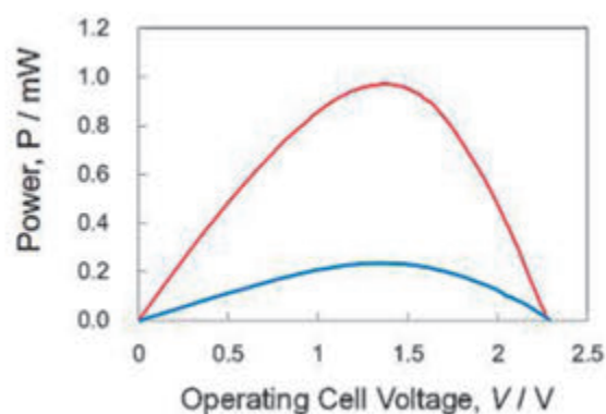
図 1.8 1x4(青)と4x4(赤)セルの出力特性
