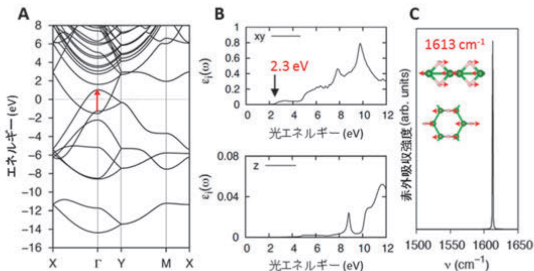
図 8 密度汎関数法で計算した図 7D で示すホウ化水素シートモデル構造の(A)バンド図、(B)光吸収スペクトル、(C)赤外吸収スペクトル
