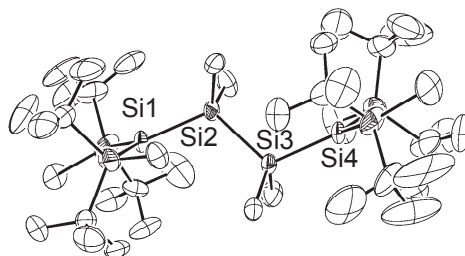
図 1・4 ジシラン連結ジ (シリルラジカル) 1 の分子構造
