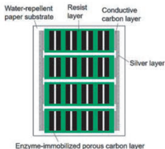
図 1.7 4x4 セルアレイの模式図
