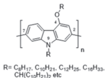
図2-1 4,9-ジ置換ポリ(2,7-カルバゾール)
