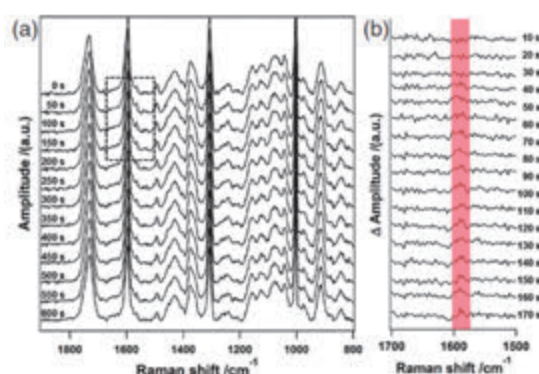
図 3-2 (a)m-TP 含有 CA フィルムの時間分解 \text{Im}[\chi^{(3)}] スペクトル、(b) 1500-1700 \text{cm}^{-1} の間の差スペクトル
