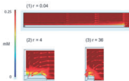
図 1.6 有限要素法によるシミュレーション
