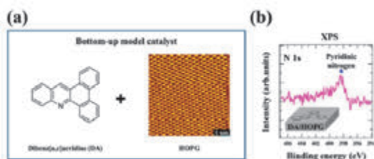
図 1 (a)ボトムアップ合成の概念図：窒素含有分子をグラファイト表面に規則的に吸着させる、(b)グラファイトにジベンゾアクリジン (DA) 分子を吸着させた表面の X 線光電子分光スペクトル、DA 分子に存在するピリジン型窒素が状態を変化させずに保たれていることが示されている。
