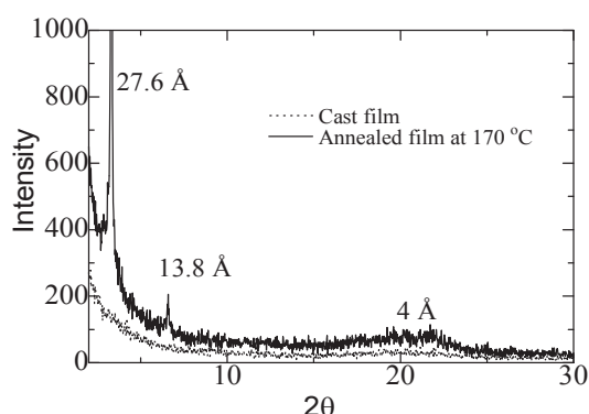
図 2-3 PDDCz キャストフィルムと熱処理サンプルの XRD パターン。
