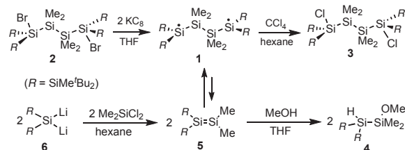
図 1・3 ジシラン連結ジ (シリルラジカル) 1 の合成および反応性
