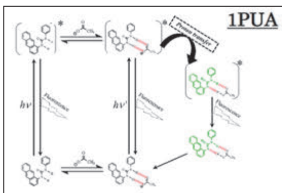
図1; 1PUA とアニオンの基底状態および励起状態における反応機構
