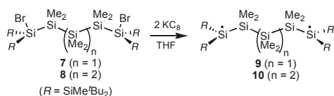
図 1・5 トリシランおよびテトラシラン連結ジ（シリルラジカル） 9 、 10 の合成
