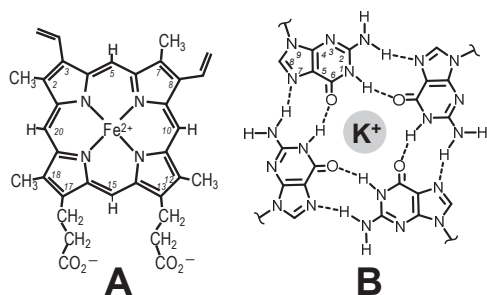
図1. ヘム(A)と G カルテット(B)の構造
