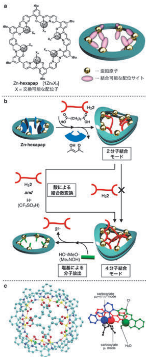
図 1 (a) 大環状亜鉛錯体 Zn-hexapap の構造 (b) 酸/塩基の刺激を用いた、多点での金属との配位結合による分子認識モードの制御 (c) X 線結晶構造解析により得られた 4 分子結合体の構造
