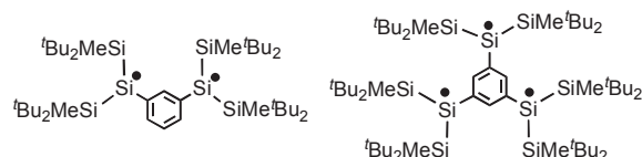
図 1・2 ベンゼン環を連結子とするオリゴ (シリルラジカル)
