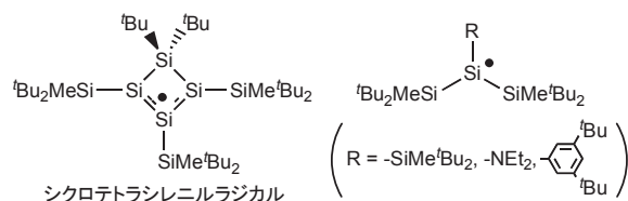
図 1・1 単離可能な安定シリルラジカル種の例
