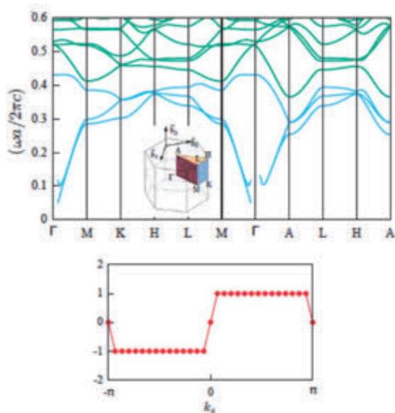
図1 ウッドパイル構造のフォトニックバンドとセクションチャーン数(大野修平氏 2018 年学位論文より引用)
