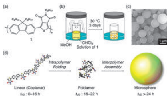
図 2 (a) \pi 共役ポリマー 1 の分子構造. (b) 蒸気拡散法による自己組織化の模式図. (c) 得られたマイクロ球体の電子顕微鏡写真. (d) 直鎖状のポリマーがフォルダマーを形成し、それらが凝集してマイクロ球体を形成する集合様式の模式図.
