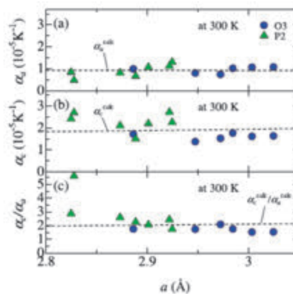
図5:層状酸化物の熱膨張係数:(a) a 軸方向 ( \alpha_a )、(b)c 軸方向 ( \alpha_c )、(c) 異方性 ( \alpha_c/\alpha_a )
