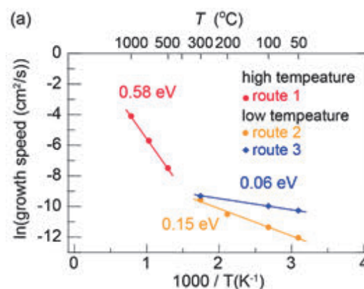
図 1-4 グラフェン成長の活性化エネルギー
