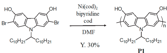
図 1-1 3,6-ジヒドロキシカルバゾールの重合
