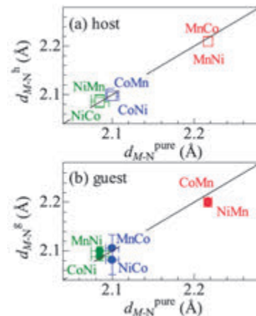
図2: PBA 中の(a)ホストおよび(b)ゲスト遷移金属周りの M-O 長。横軸はゲスト遷移金属しか含まない層状酸化物の M-O 長。
