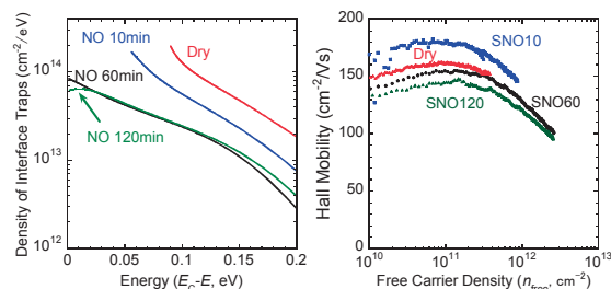
図 3 伝導帯近傍の界面準位密度とホール移動度の可動キャリア密度依存性
