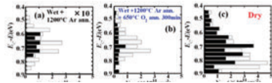
図1 界面準位密度分布。(a) ウェット酸化膜、(b) 酸素中の追加熱処理がされたウェット酸化膜、(c) 乾燥酸素酸化膜
