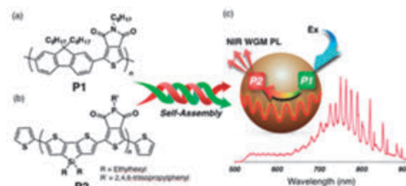
図 3 (a, b) エネルギー供与性ポリマー P1 とエネルギー受容性ポリマー P2 の分子構造. (c) 球体内 FRET を介した近赤外 WGM 発光スペクトルと模式図.
