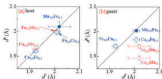
図1: ペロブスカイト酸化物中の(a)ホストおよび(b)ゲスト遷移金属周りの M-O 長。横軸はゲスト遷移金属しか含まない層状酸化物の M-O 長。
