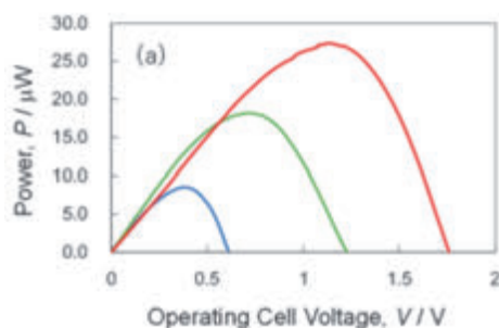
図 1.5 片面に印刷された電池の直接接続 青 単セル, 緑 2 直列接続, 赤 3 直列接続
