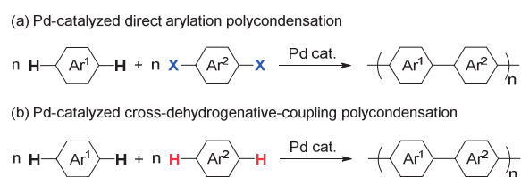
Scheme 1 (a)直接的アリール化重合と(b)脱水素型クロスカップリング重合
