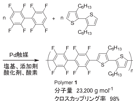
Scheme 2 脱水素型クロスカップリングによる Polymer 1 の合成
