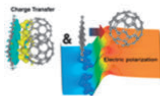
図 1・1 図 1:C60 分子膜とグラフェンからなる vdW ヘテロ構造における電荷移動と分極
