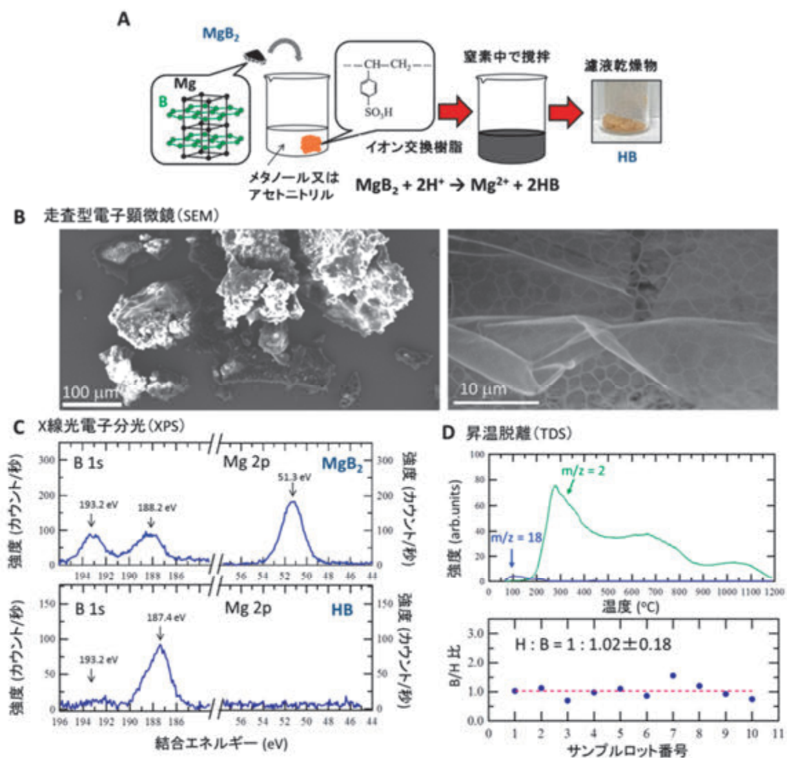
図 5 ホウ化水素(HB)シートに関する(A)生成方法の模式図、(B)走査型電子顕微鏡像、(C)X線光電子分光スペクトル、(D)昇温脱離測定結果と算出した B/H 比
