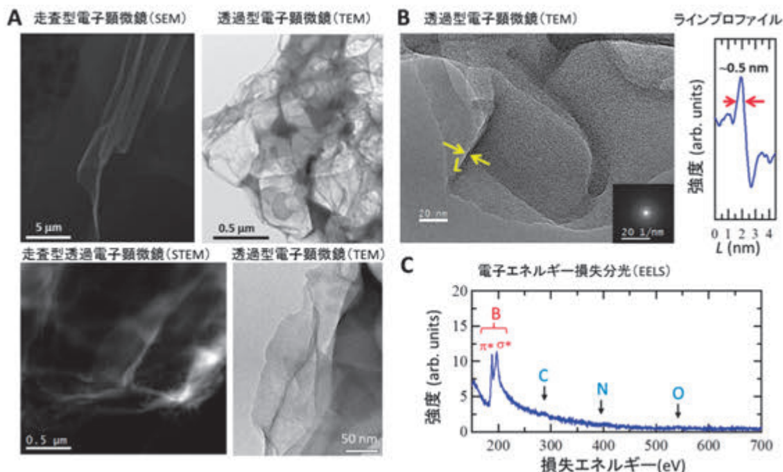
図 6 ホウ化水素(HB)シートの(A)走査型電子顕微鏡像、透過型電子顕微鏡像、および走査型透過電子顕微鏡像、(B)透過電子顕微鏡像とラインプロファイル、(C)電子エネルギー損失分光スペクトル
