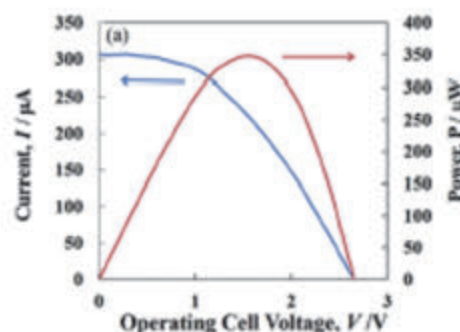
図 1.3 アレイ型電池の出力特性
