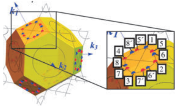
図2 ダイヤモンド格子上の力学系のワイル点の対生成、対消滅 (Y. Takahashi, T. Kariyado, Y. Hatsugai "Weyl points of mechanical diamond", arXiv: 1801.06784 )
