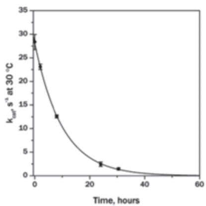
図 3.2 ヒドロゲナーゼの溶液中での酵素の安定性
