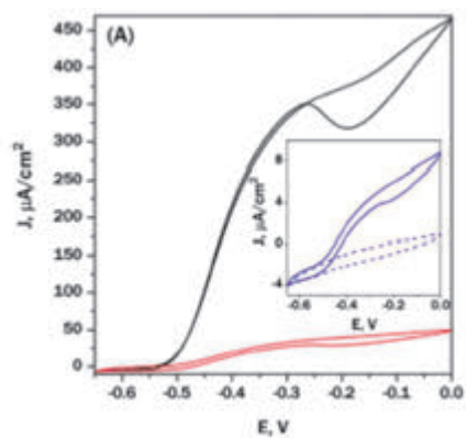
図 3.1 ヒドロゲナーゼによる水素酸化
