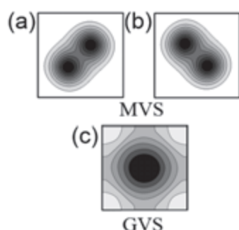
図2：正方形薄膜超伝導体の渦度 L=2 の渦糸状態。(クーパー対密度の等高線表示。黒が中心核。) (a)(b)多重渦糸状態、(c)巨大渦糸状態。
