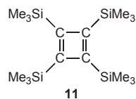
図 2・1 シリル置換シクロブタジエン
