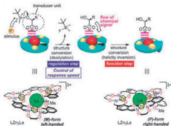
図 2 シロキシカルボン酸イオンの脱シリル化を制御段階とする人工のらせん反転システム
