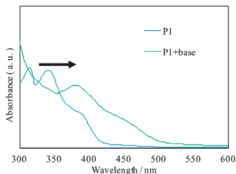
図 1-3 DMSO 中の P1 の紫外可視吸収スペクトルと塩基添加効果
