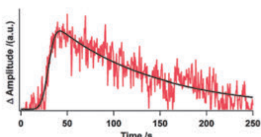
Fig.3 OH変角振動の振幅の時間的プロファイル(赤)、フィッティング曲線(黒)
