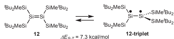
図 2・3 シリル置換ジシレン 12 における熱励起平衡
