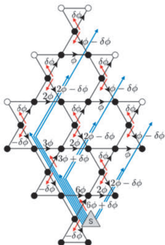
図4 格子上でランダウ準位に射影した擬ポテンシャルを構成するためのストリングゲージ:カゴメ格子の例 (K. Kudo, T. Kariyado, Y. Hatsugai, " Many-Body Chern Numbers of \nu=1/3 and 1/2 States on Various Lattices", J. Phys. Soc. Jpn. 86, 103701 (2017))
