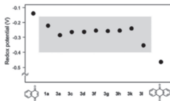
図 2.2 キノ誘導体の酸化還元電位
