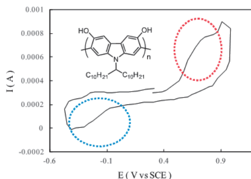
図 1-2 P1 のサイクリックボルタンモグラム
