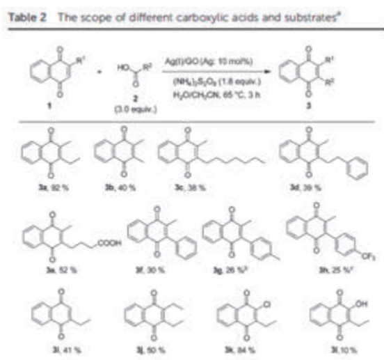
図 2.1 基本的な合成スキームと今回合成したキノ誘導体
