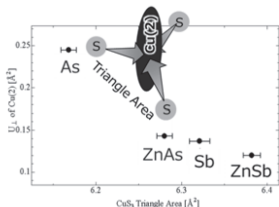
図2 S 3 三角形面積と熱振動の関係
