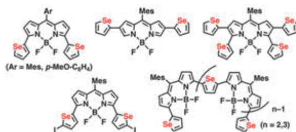
図 3 セレンオフェン環を有する BODIPY 単量体および鎖状多量体
