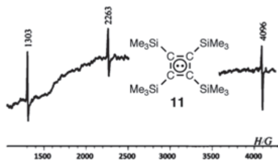
図 2・2 395 K におけるシリル置換シクロブタジエン 11 の励起三重項状態の EPR スペクトル ( \Delta M_S = \pm 2 , 1303 G; \Delta M_S = \pm 1 , 2263, 4096 G)
