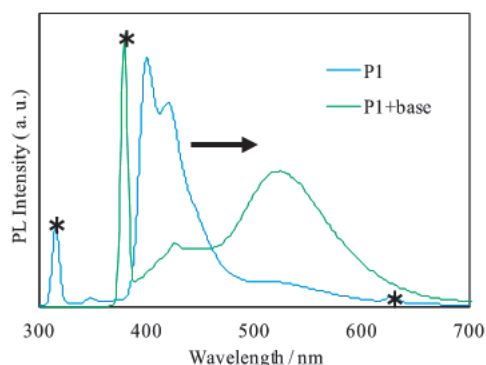
図1-4 DMSO中のP1の蛍光スペクトルと塩基添加効果
