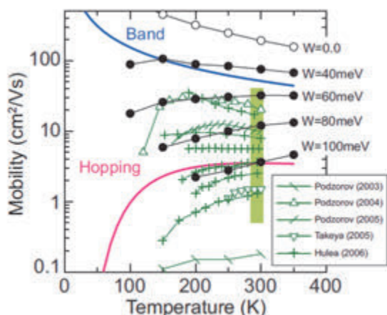
図 2-1 ルブレン結晶の移動度理論 Phys. Rev. B 95, 035433 (2017)
