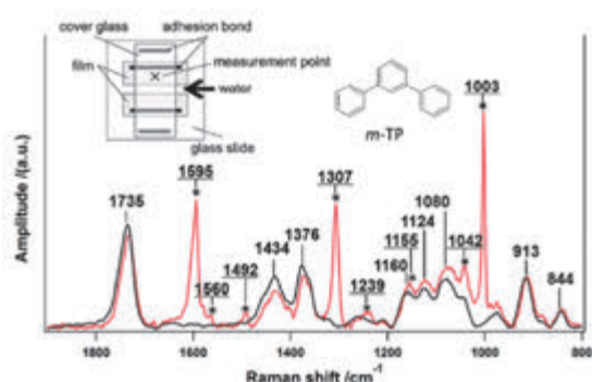
図 3-1 m-TP 含有 (赤)、非含有 (黒) CA フィルムの \text{Im}[\chi^{(3)}] スペクトル
