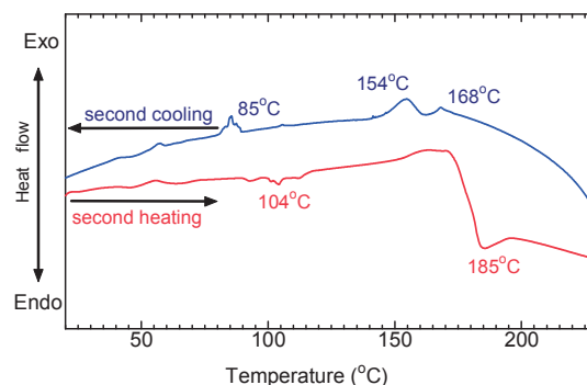
図2-2 PDDCz のDSC 結果 .
