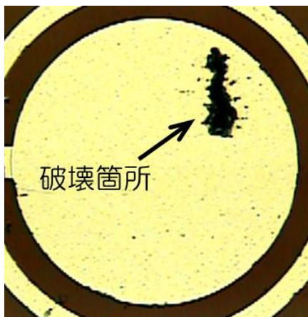
図 1.322MeV-Kr イオン入射により破壊した SiC MOS キャパシタの顕微鏡写真
